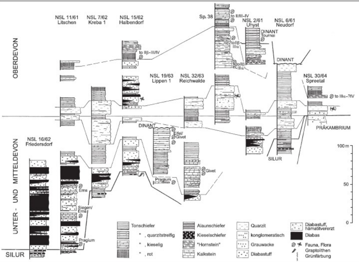
Abb. 2.10-4. Vereinfachte stratigraphische Säulenprofile zum Aufbau des Devon im Görlitzer Schiefergebirge (BRAUSE 1965).
